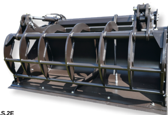
GRL.S.2E Grappin dents soudées 2 ébauches dents affleurantes
